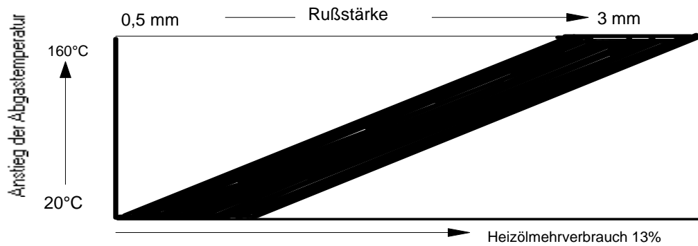
Bild 2: Zusammenhang zwischen Rußstärke und HEL-Mehrverbrauch
